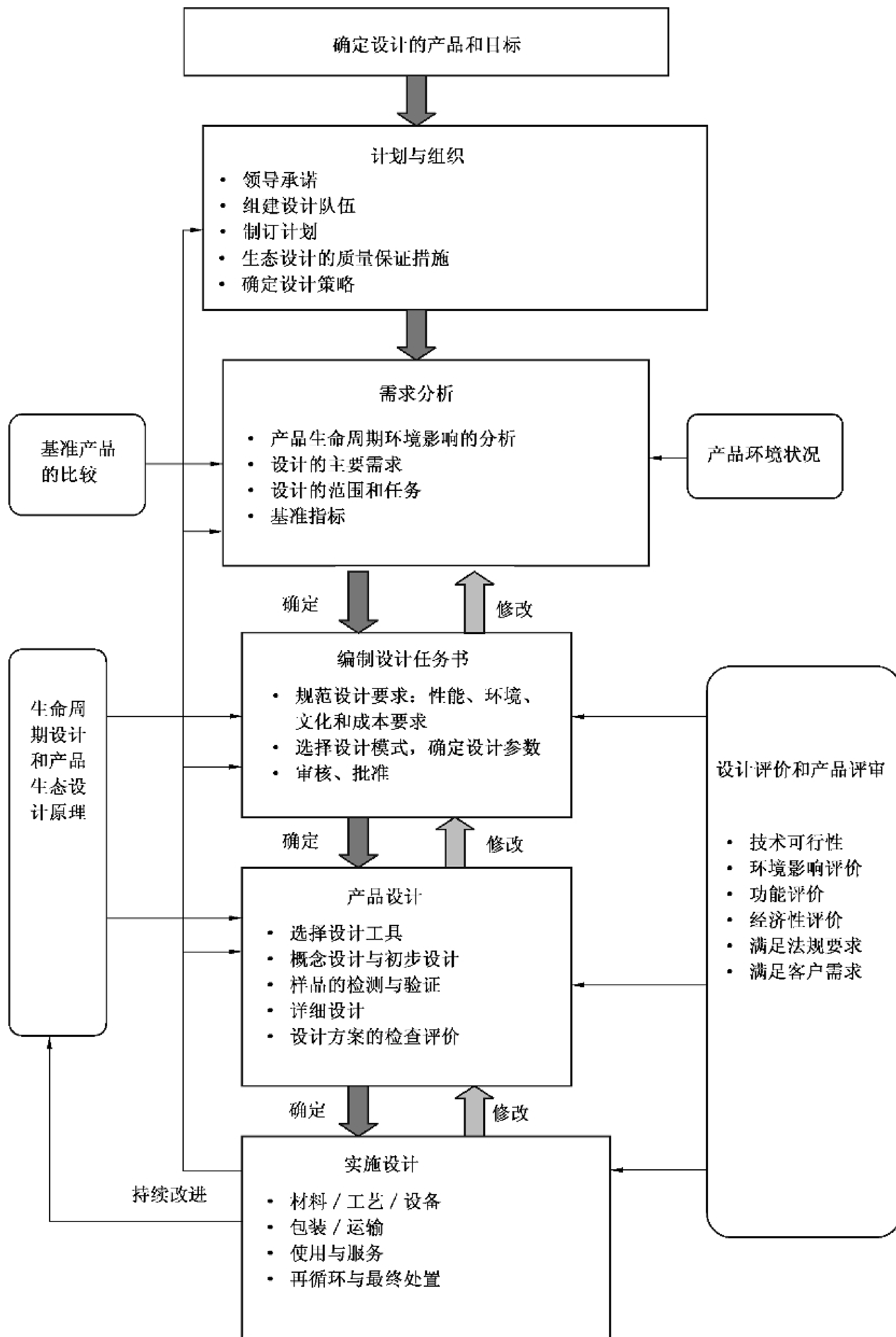
图 2 产品生态设计过程示意图
